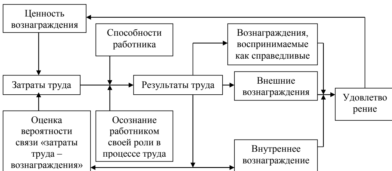
Рис. 7.3. Модель Портера-Лоулера
