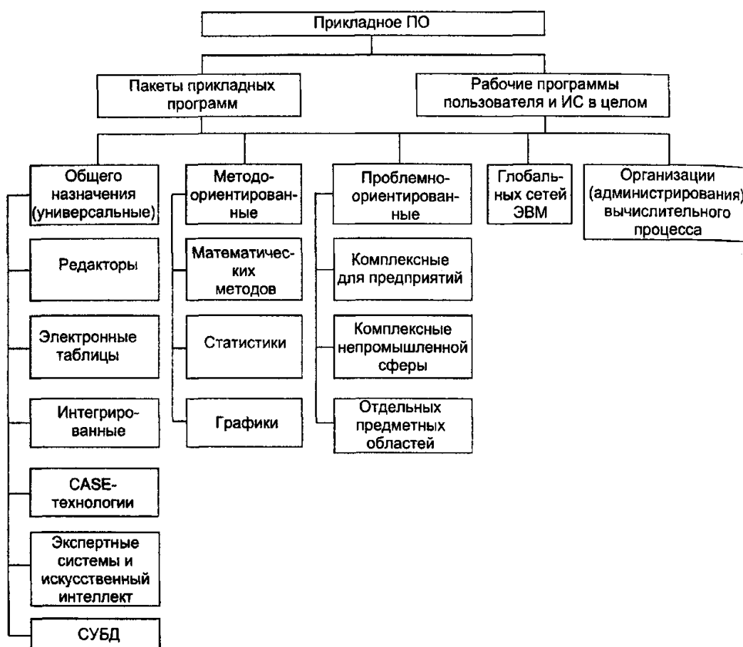
Рис. 3.1. Прикладное программное обеспечение
