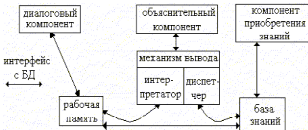
Рис. 6.3. Структура статических ЭС
