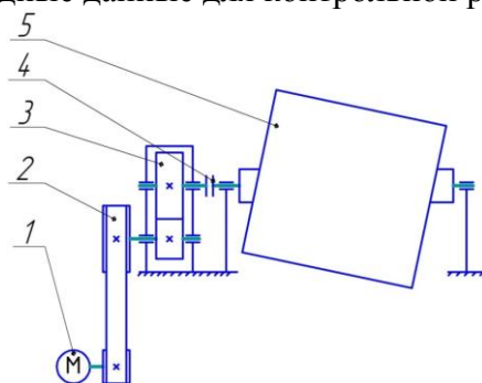
1 – электродвигатель, 2 - ременная передача, 3 – редуктор, 4- муфта, 5 –галтовочный барабан Рисунок 1- Кинематическая схема привода
