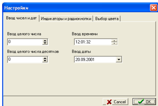
Рисунок 6.2 – Страница «Ввод чисел и дат»
