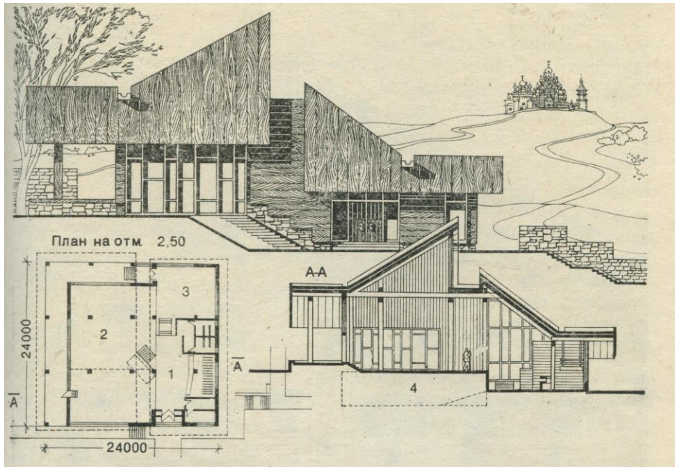
Музей народного творчества в Кижях, запроектированный из дерева: 1 – вестибюль; 2 – большой выставочный зал; 3 – малый зал; 4 - хранилище
